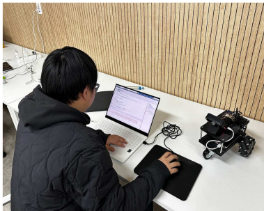
아두이노 코딩
